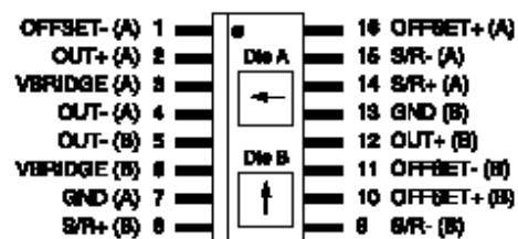
HMC1022
