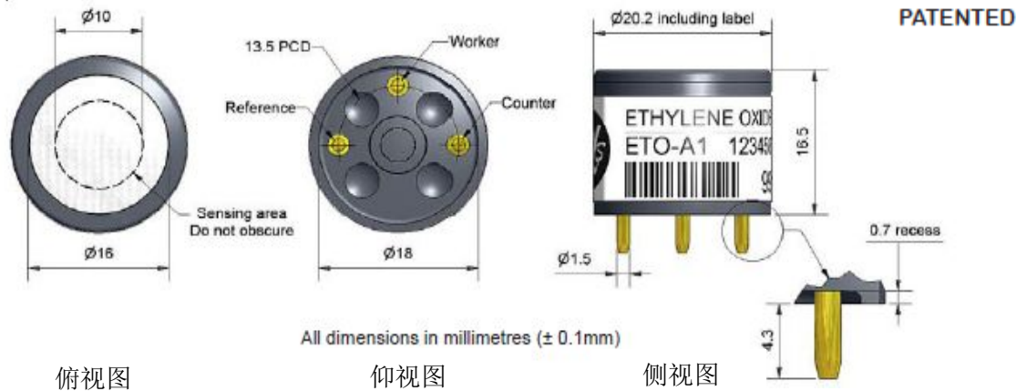
图1 ETO-A1 示意图
