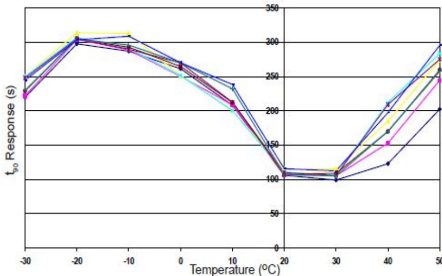
图4 响应时间温度特性
