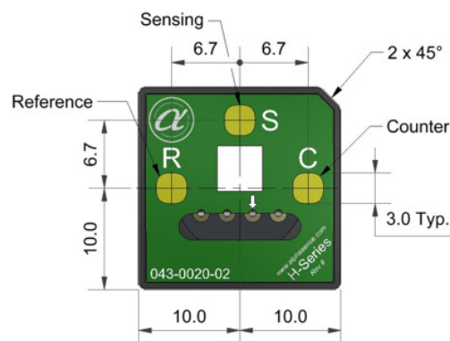
底视图
