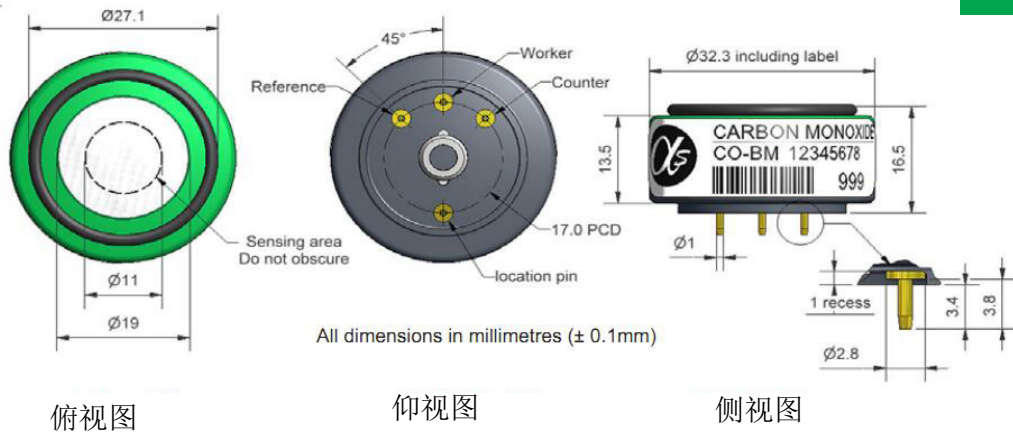
图1 CO-BM示意图
